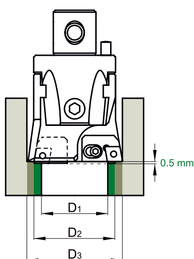
Mandrilagem escalonada
