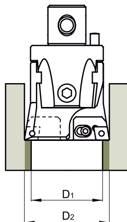
Mandrilagem simétrica
