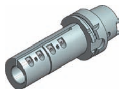
geschlitzter Bohrstangenhalter Slotted boring bar holder
